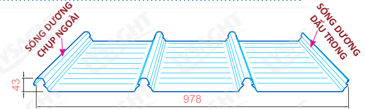
Hình 5.3.2.a Tôn Lysaght® Klip-lok® Optima®
