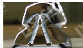
Hình 5.3.3.2.b Đai KL98 đã cài vào tôn
