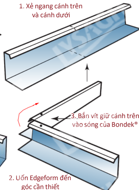
Hình 7.4.2.b Bề tấm viền cho góc trong sàn
