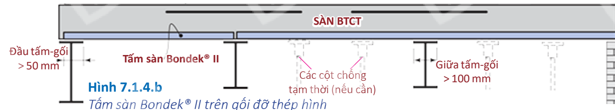
Hình 7.1.4.a Tấm sàn Bondek® II trên gổ đỡ bê tông
