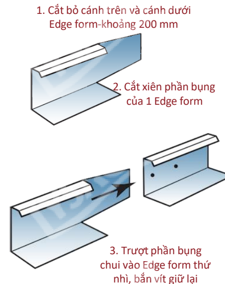
Hình 7.4.2.c Nối 2 tấm viền cạnh
