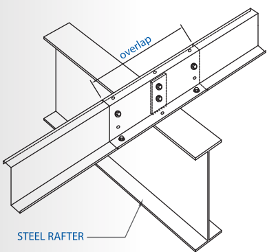
Liên kết có bản mã / Cleat Connections
