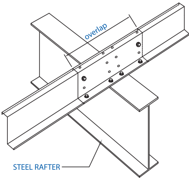
Liên kết không có bản mã / Cleatless Connections
